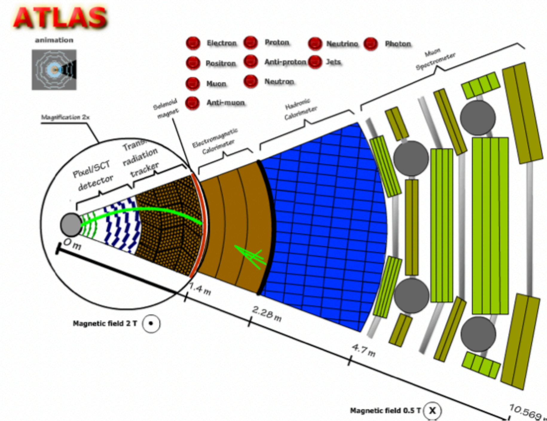
positron
