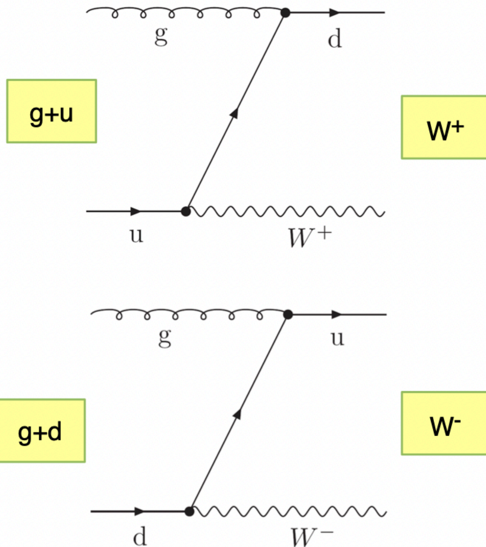
zderzenia kwark-gluon
